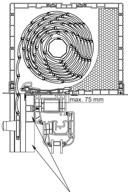
Listwa dystansowa
