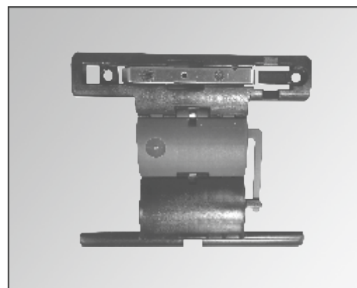
WBZ2-40 WIESZAK BLOKADA ZACZEPOWY 2-częściowy do rury oktagonalnej 40 mm
