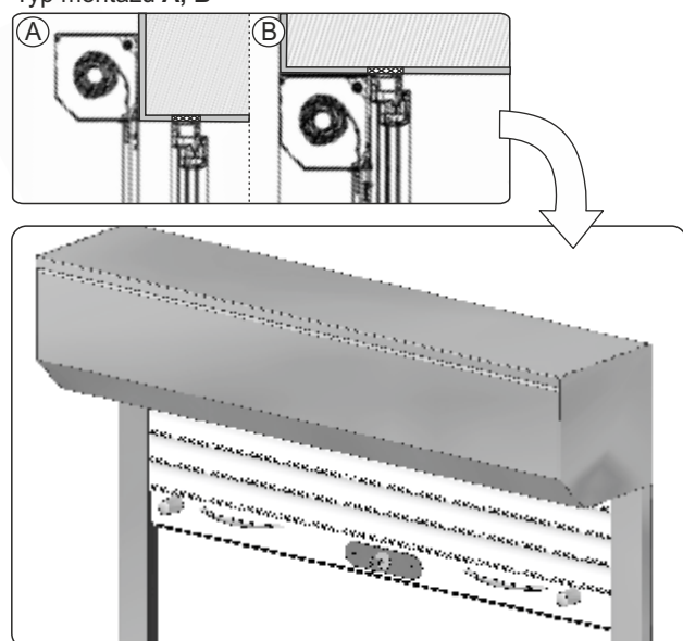
Typ montażu A, B
