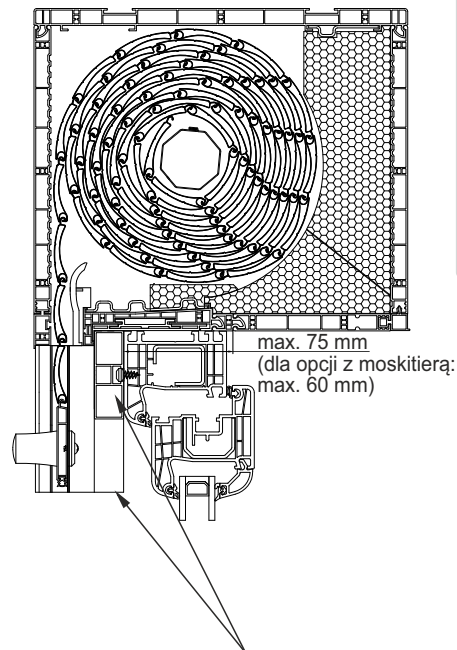
Listwa dystansowa
