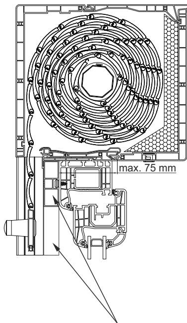
Listwa dystansowa
